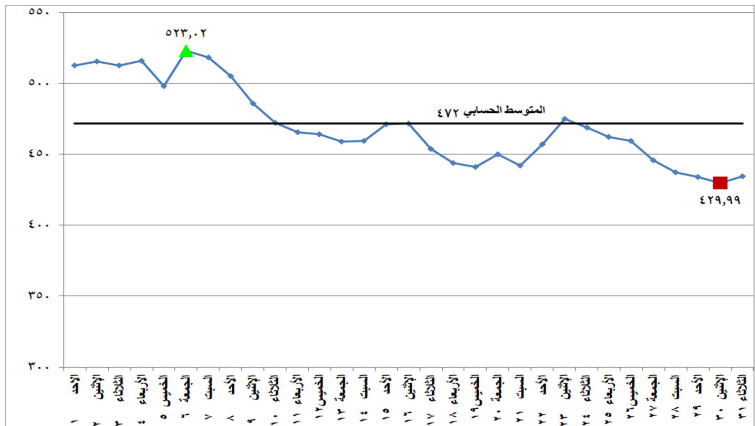
شكل (١٤) معامل انبعاثات غاز ثاني اكسيد الكربون المكافئ على مدى شهر أغسطس ٢٠٢١
