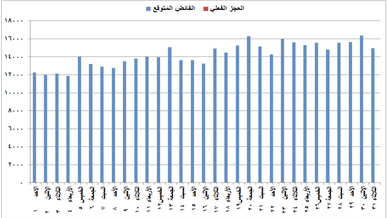
شكل (٧) الفائض والعجز المتوقع للقدرات خلال شهر أغسطس ٢٠٢١
