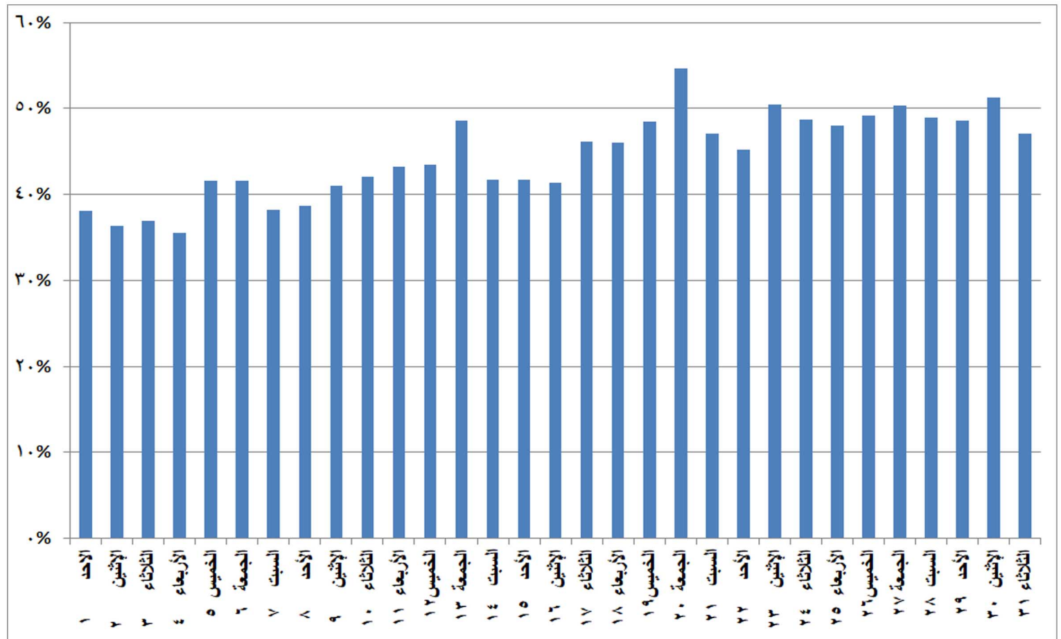
شكل (٢٨) نسب الفائض للحمل الاقصى المسجل يوميا خلال شهر أغسطس ٢٠٢١
