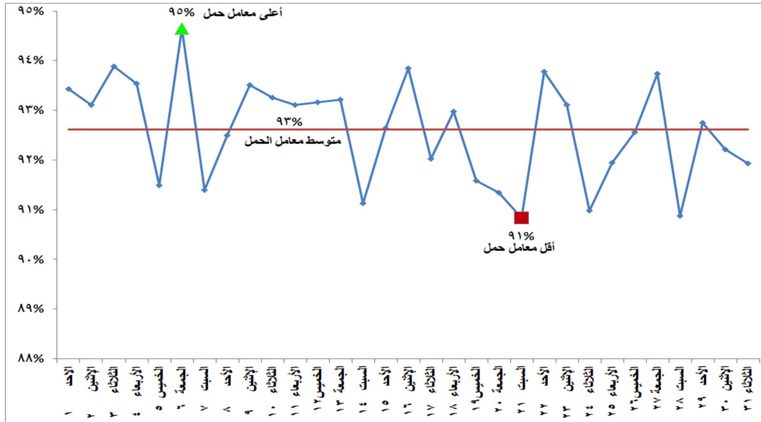
شكل (١٢) إجمالي معامل الحمل لوحدات الانتاج خلال شهر أغسطس ٢٠٢١
