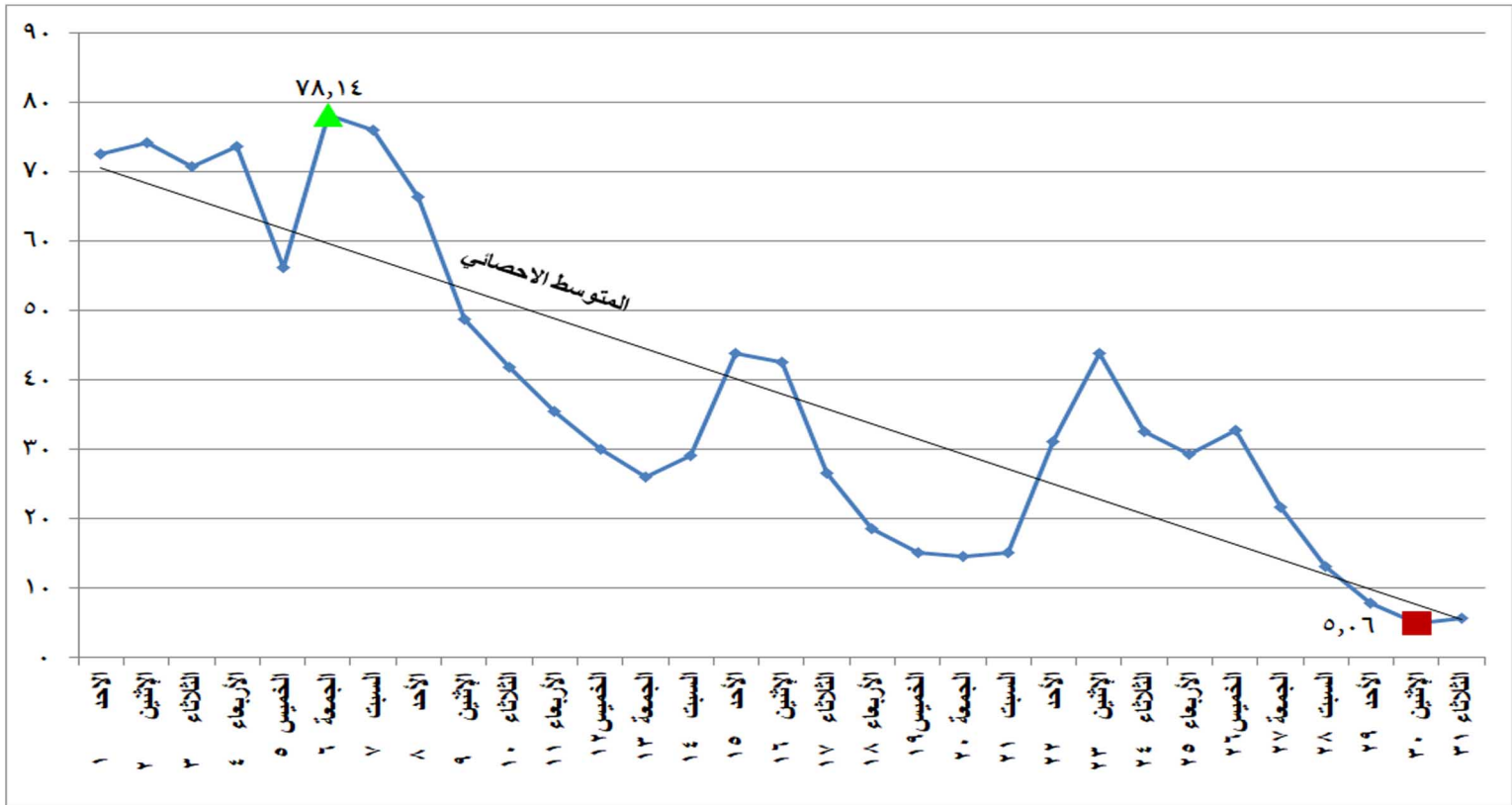
شكل (١٩) الطاقة الكهربائية المنتجة من المازوت خلال شهر أغسطس ٢٠٢١
