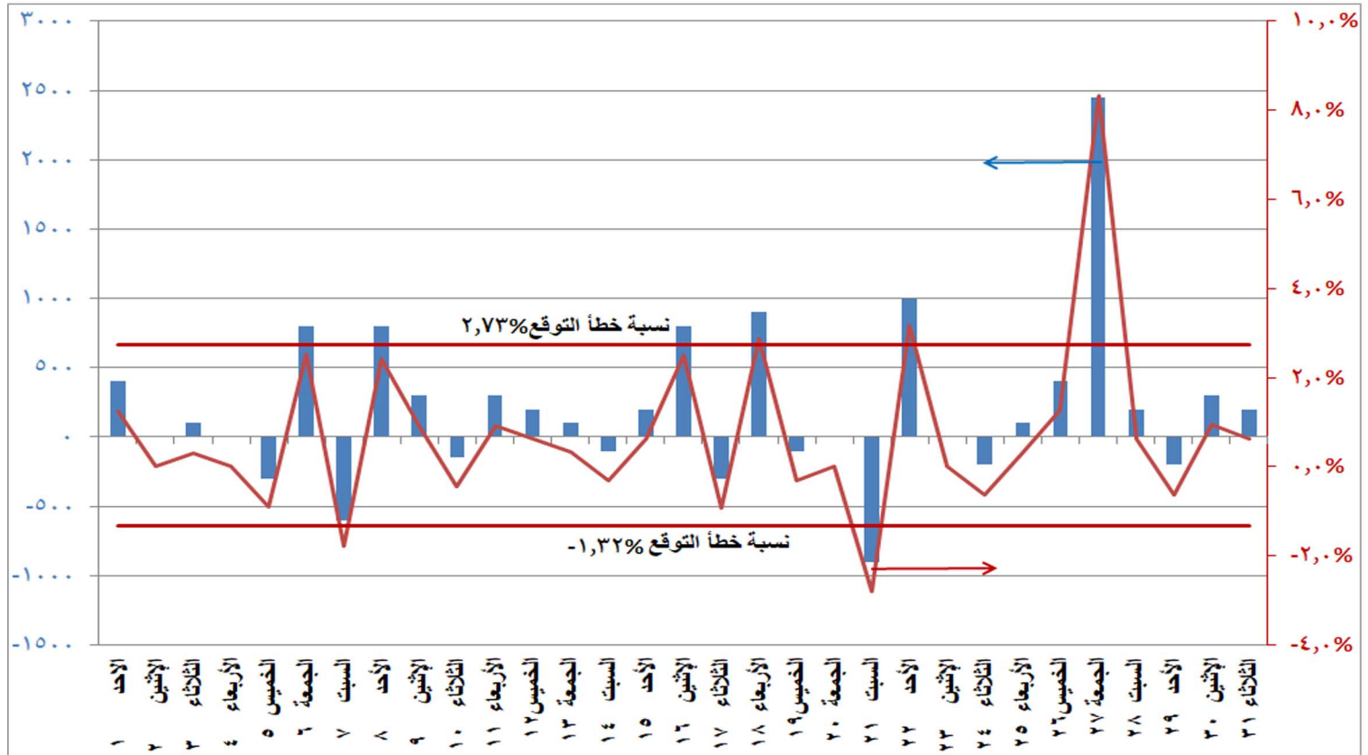
شكل (١٠) الفرق بين الحمل الأقصى المتوقع والمسجل فعليا ونسبة الفرق إلى الحمل المسجل فعليا خلال شهر أغسطس ٢٠٢١
