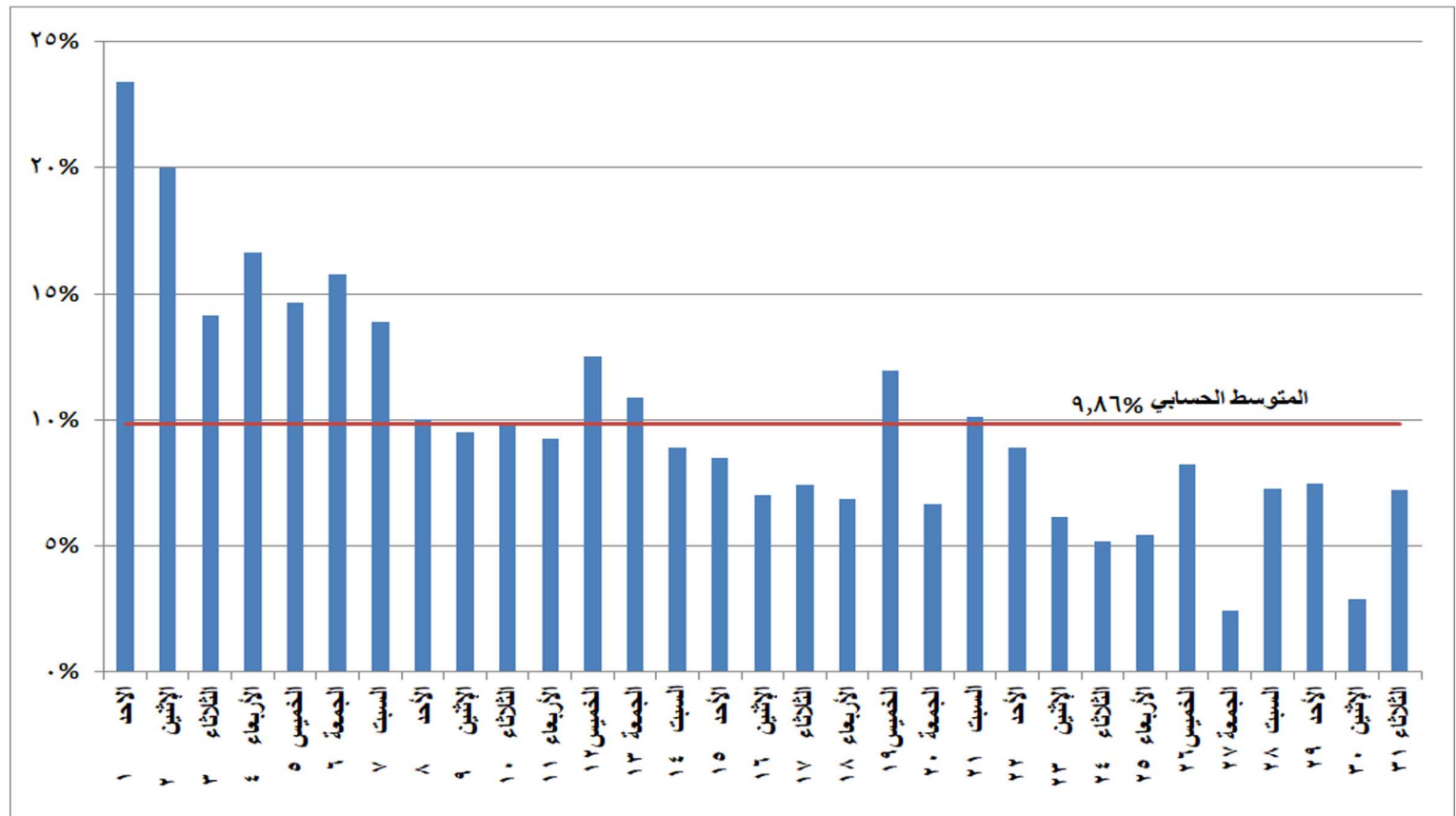
شكل (١٦) نسب التغير في الطاقة الكهربائية المنتجة خلال شهر أغسطس ٢٠٢١ مقارنة بالشهر المماثل من العام السابق
