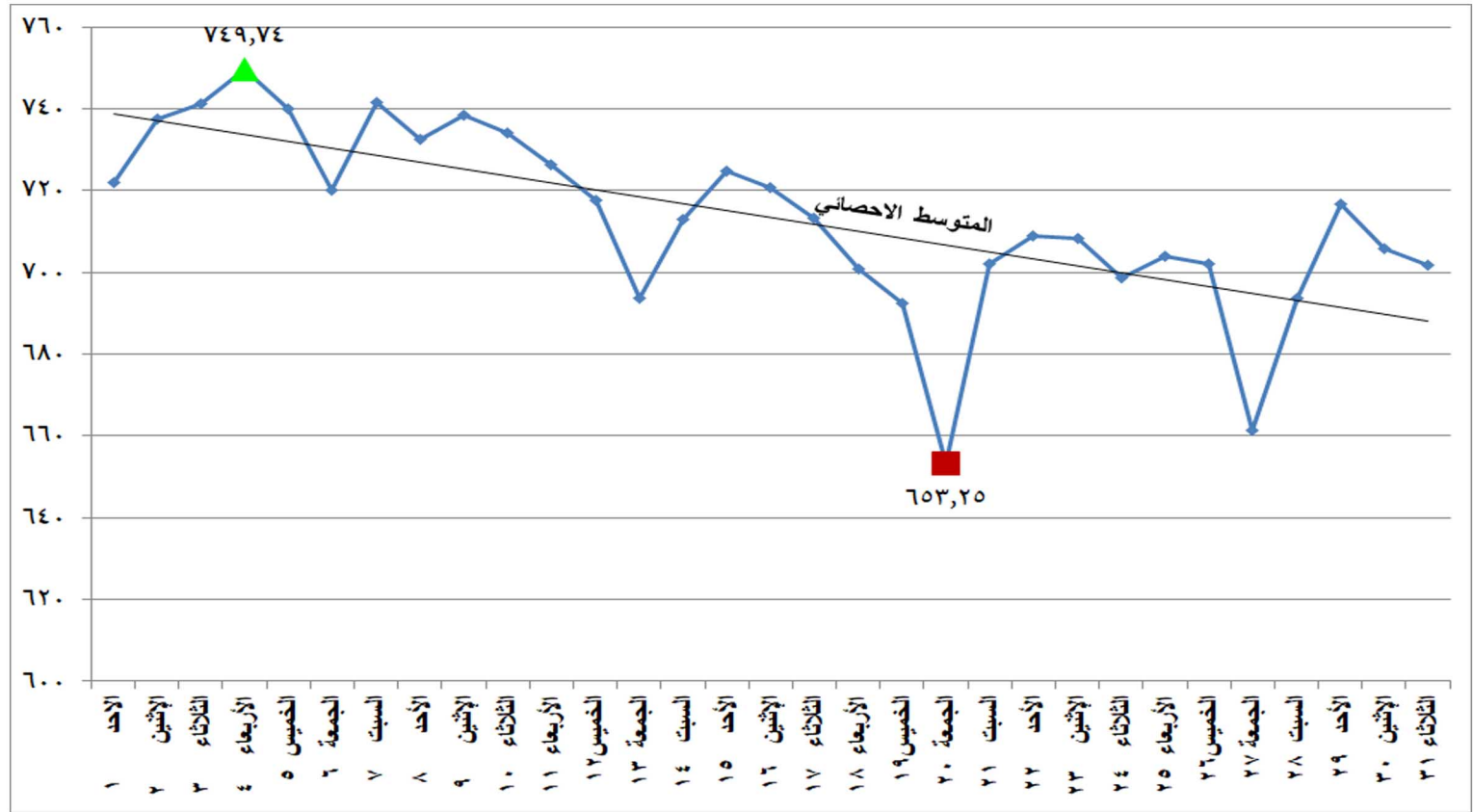
شكل (١٥) إجمالي الطاقة الكهربائية المنتجة من كل المصادر الأولية خلال شهر أغسطس ٢٠٢١
