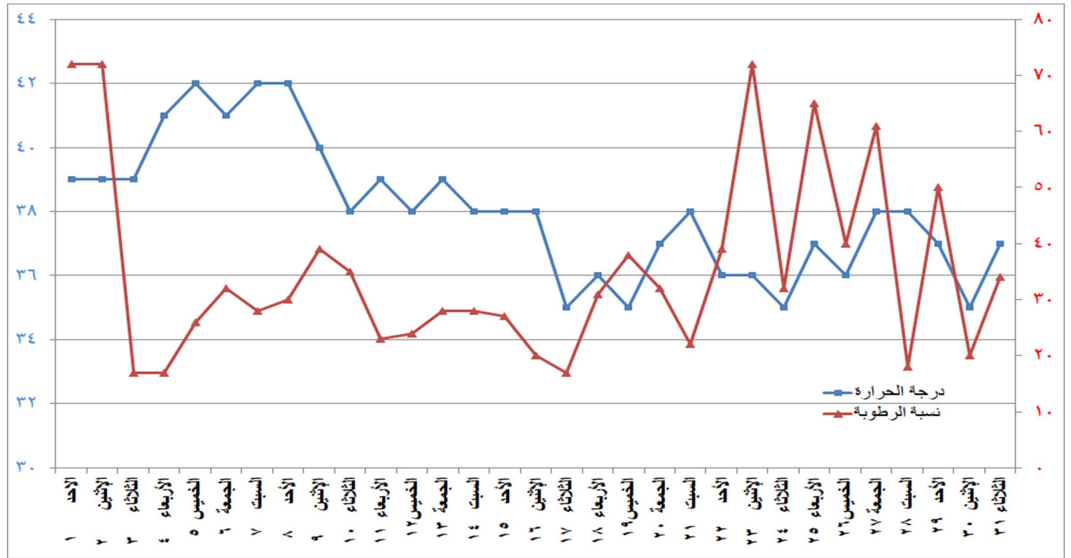
شكل (١١) التغيير في درجة الحرارة والرطوبة النسبية خلال شهر أغسطس ٢٠٢١
