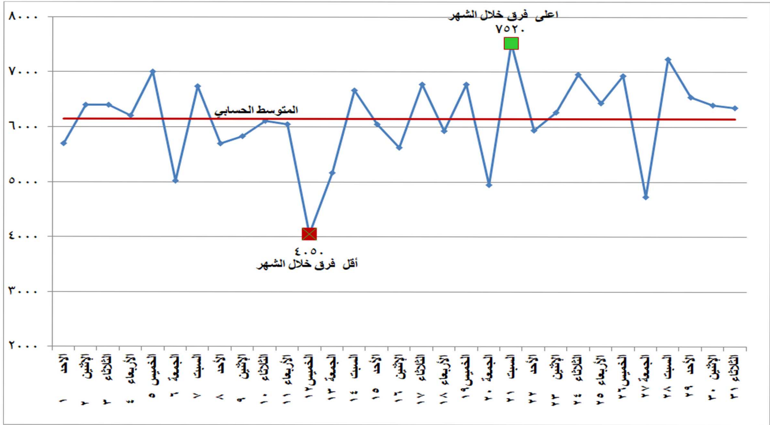
شكل (٣) الفرق بين أقصى وأدنى حمل خلال شهر أغسطس ٢٠٢١
