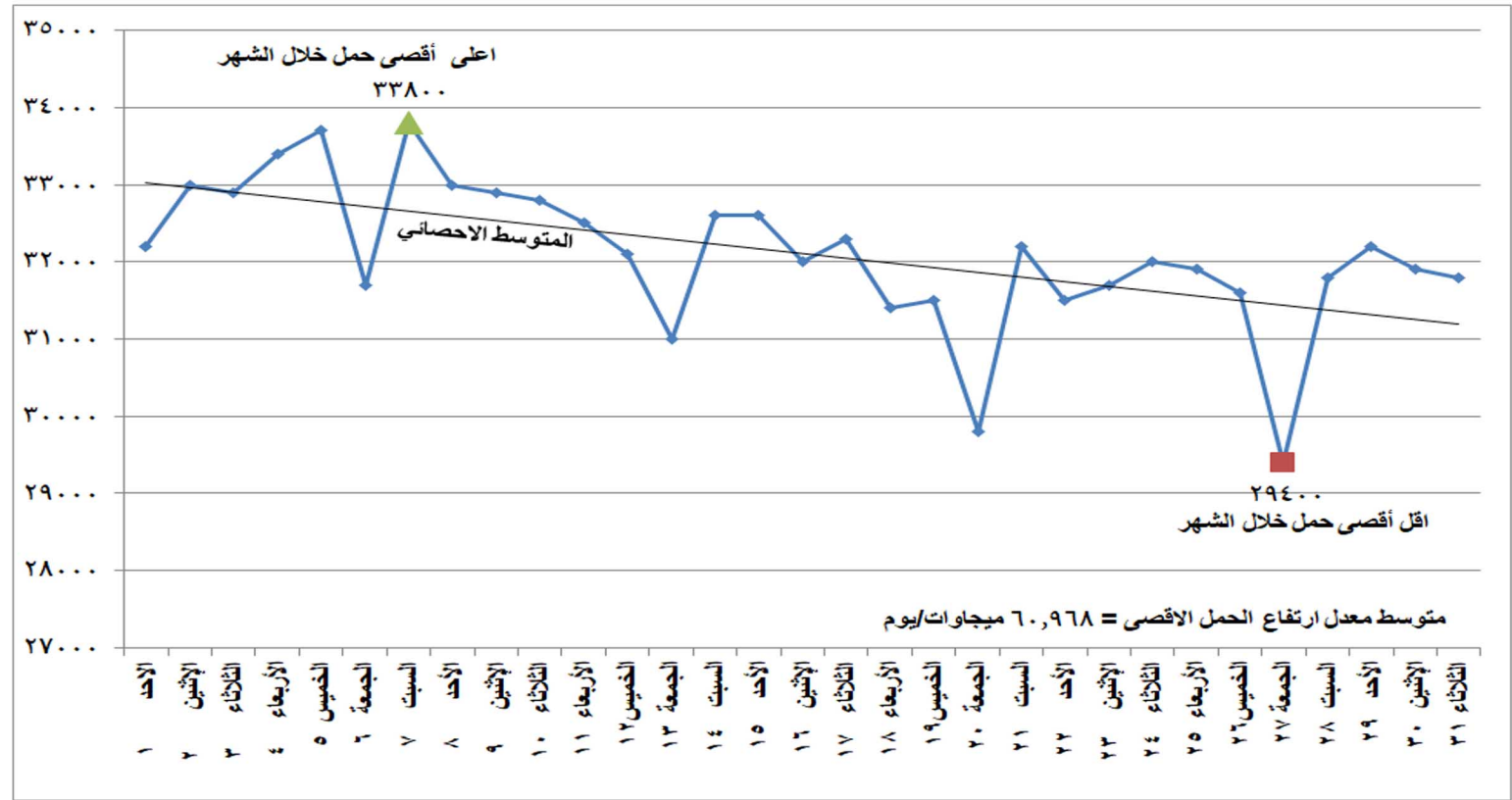
شكل (١) تطور الحمل الاقصى اليومي خلال شهر أغسطس ٢٠٢١
