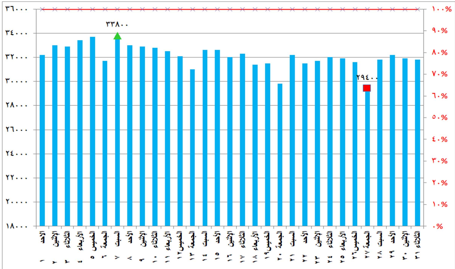
شكل (٥) قدرات الانتاج المتاحة ونسبتها للحمل الأقصى خلال شهر أغسطس ٢٠٢١
