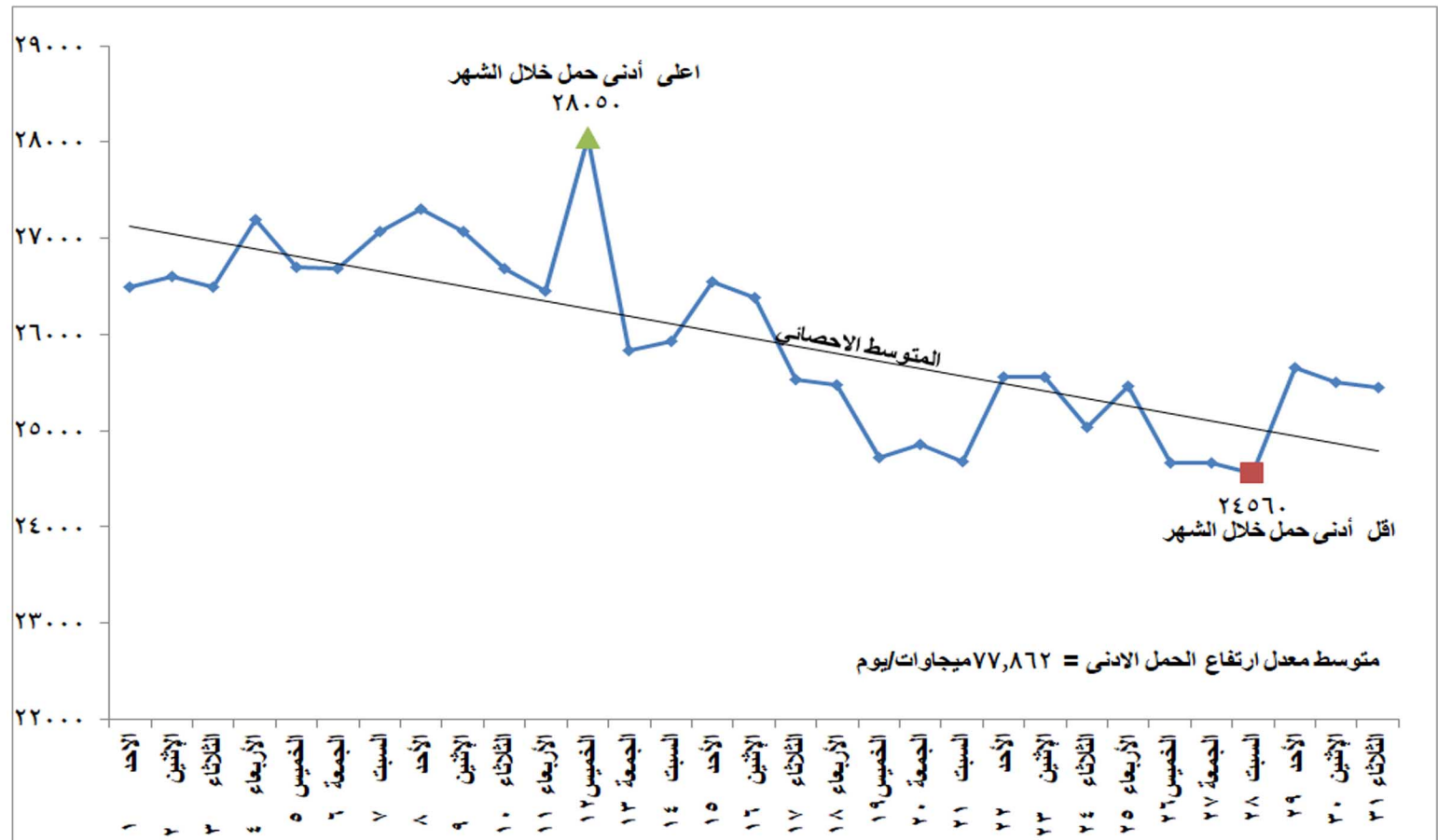
شكل (٢) تطور الحمل الادنى اليومي خلال شهر اغسطس ٢٠٢١
