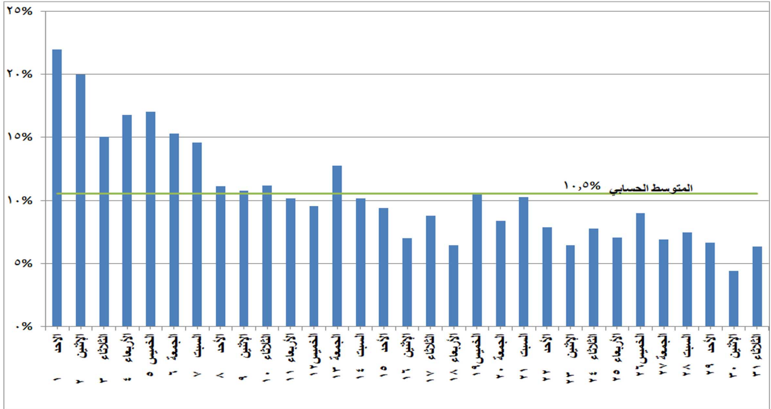
شكل (٩) النسب المئوية للتغير في الحمل الاقصى خلال شهر أغسطس ٢٠٢١ مقارنة باليوم المماثل من العام الماضي
