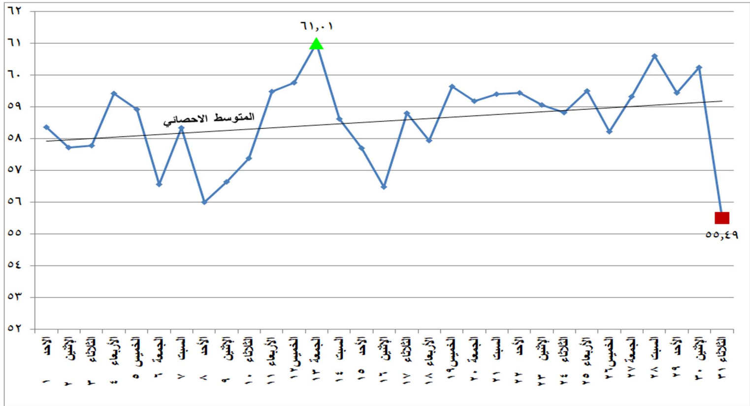
شكل (٢٣) الطاقة الكهربائية المنتجة من المصادر المائية خلال شهر أغسطس ٢٠٢١
