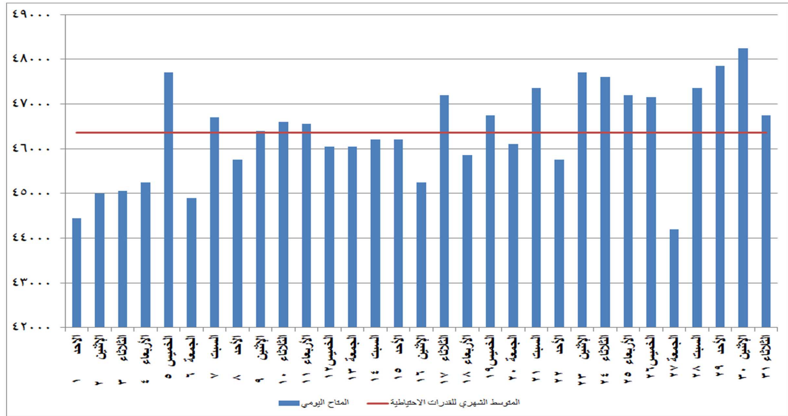
شكل (٢٧) القدرات المتاحة يوميا والمتوسط الشهري للقدرة الاحتياطية خلال شهر أغسطس ٢٠٢١
